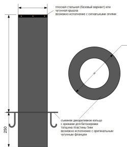
ТИП 1 под бетонирование
