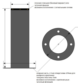
ТИП 2 - анкерное крепление
